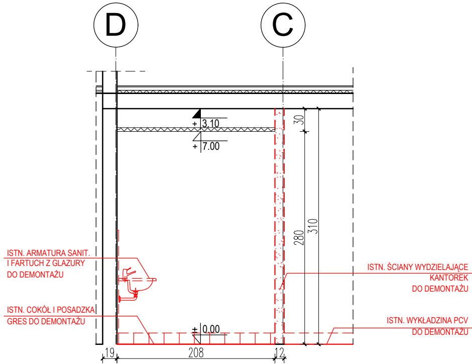
POM. 1.15- WIDOK A-A
