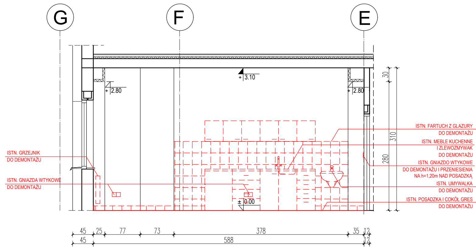
POM. 1.26- WIDOK A-A
